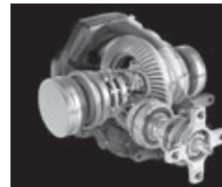
AMG Hinterachs-Sperrdifferenzial
